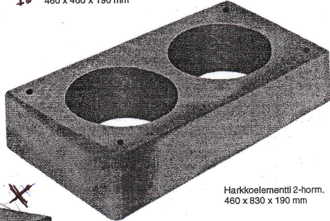
1. Harkkoelementti 460 x 460 x 190 mm
